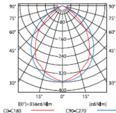
krzywa rozsyłu światłości / curve of intensity distribution \eta = 75\%
